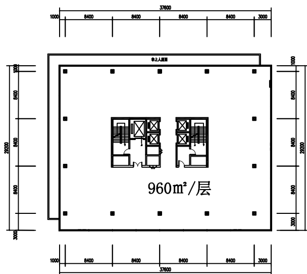
八、九层平面图
