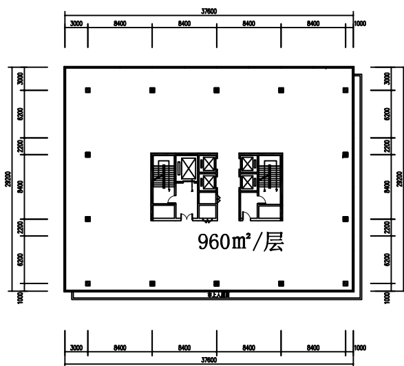
十二层平面图
