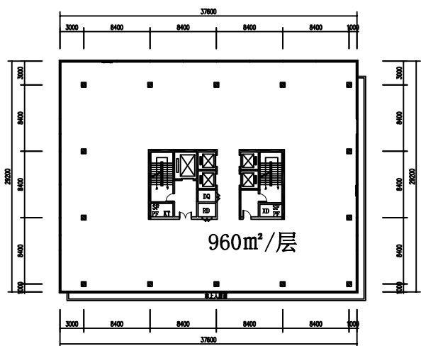
六、七层平面图
