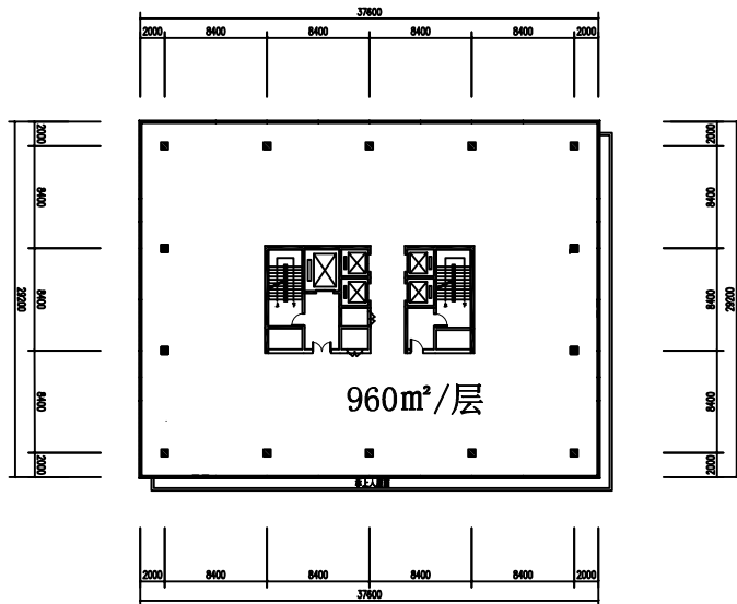
十、十一层平面图
